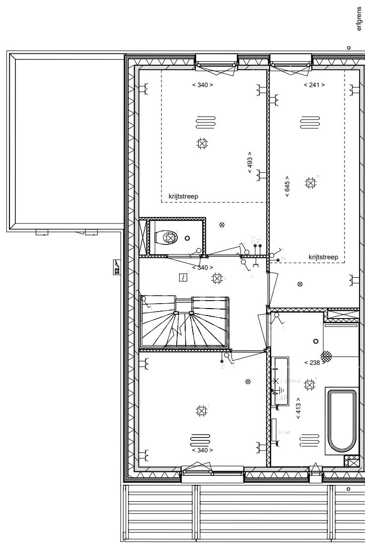
eerste verdieping
