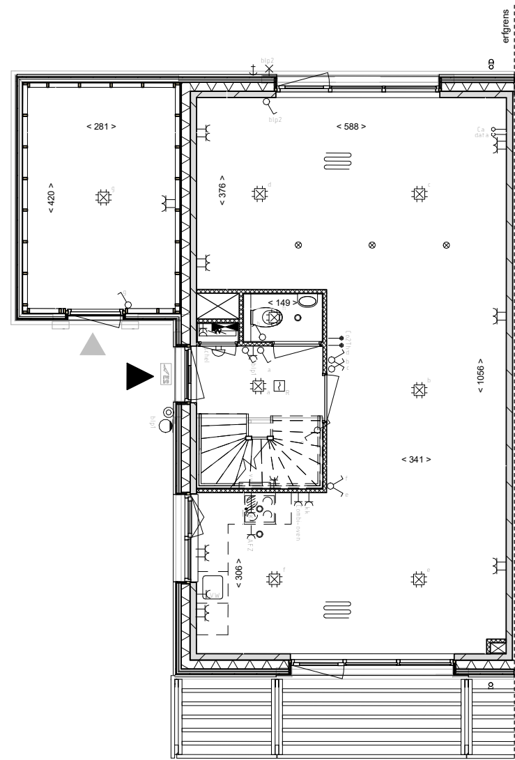
begane grond
